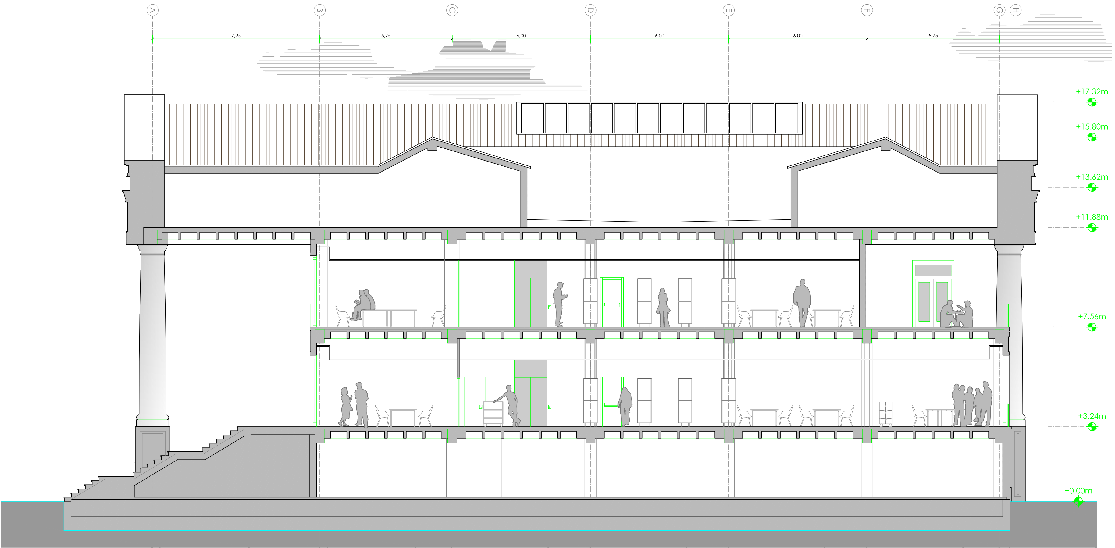
BIBLIOTECA - SECCIÓN TRANSVERSAL B-B'
