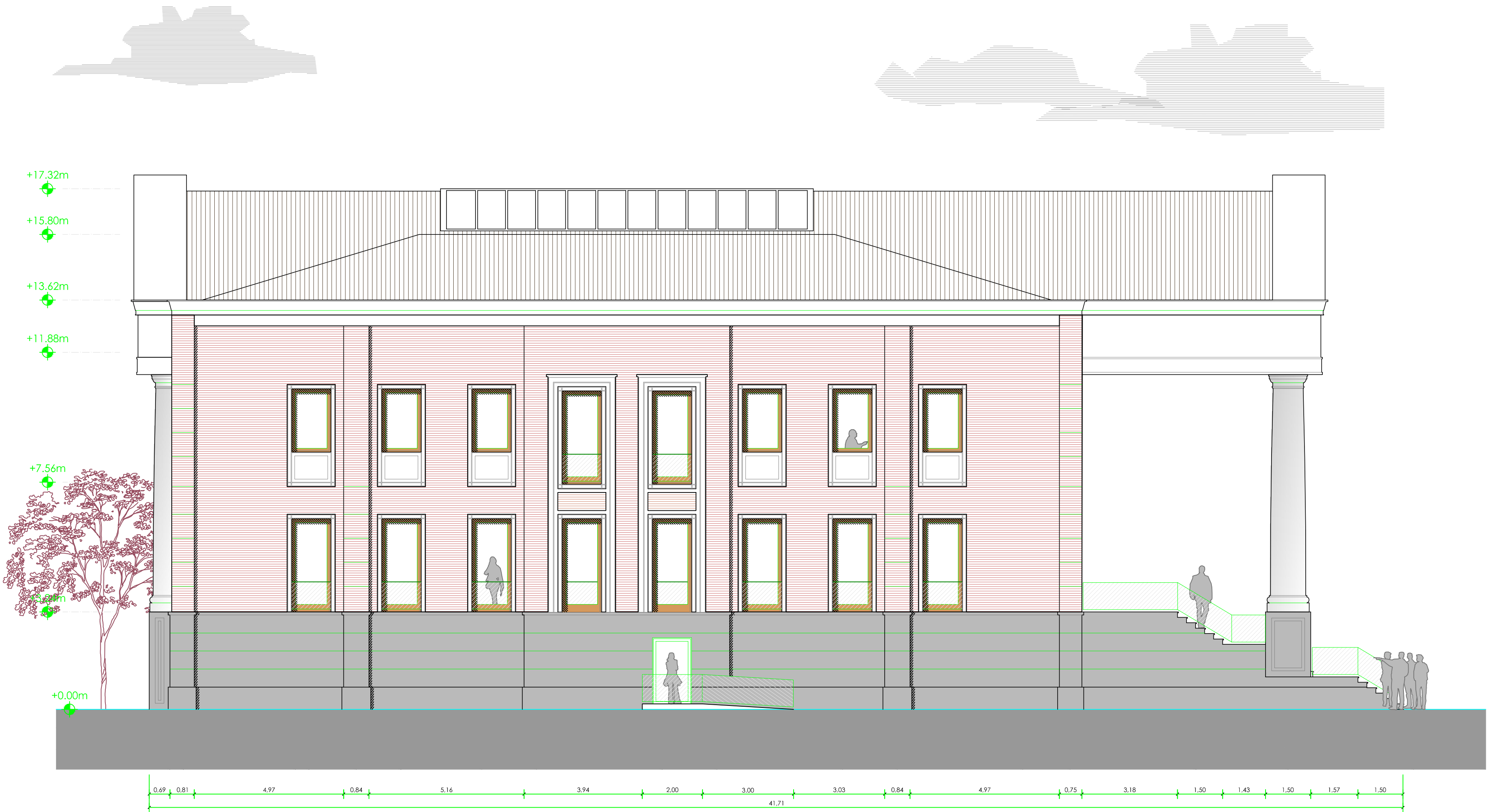
BIBLIOTECA - ALZADO NORTE
