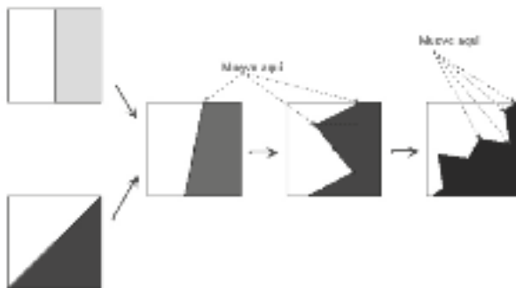
Figura 7. Transformación generalizada
