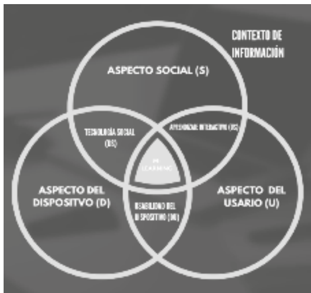
Figura 6. Modelo Frame
